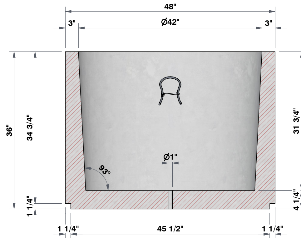
SECTION A-A 7/8"=1'
