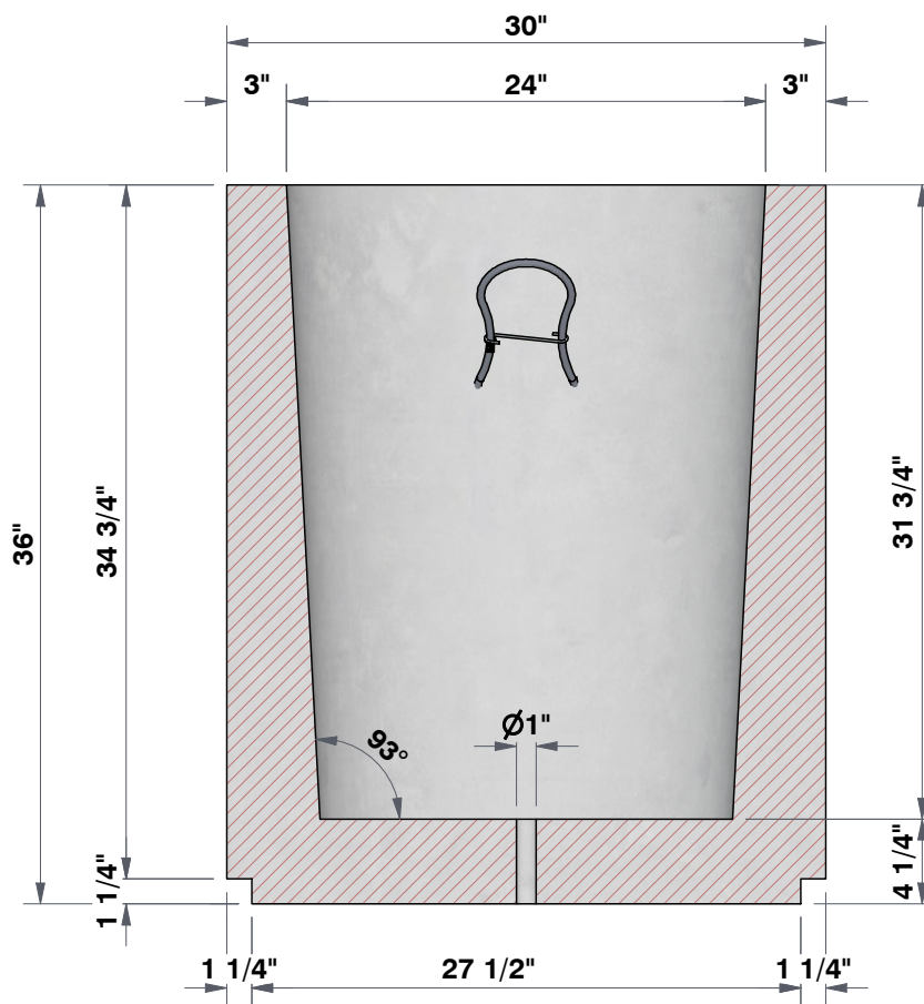
SECTION A-A 1 1/8"=1'
